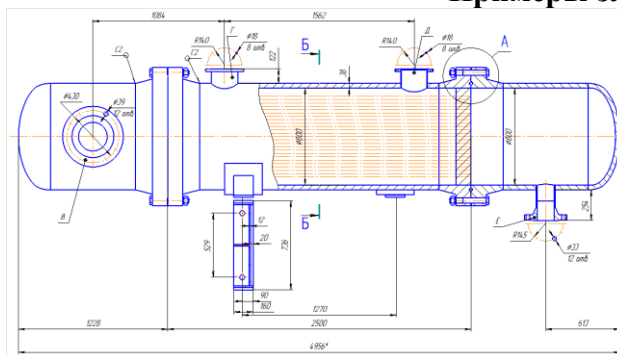
Холодильник-конденсатор
